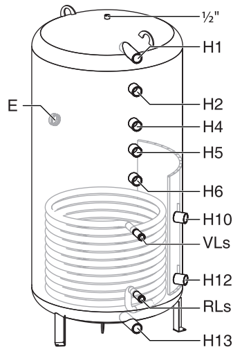
BS 500, 750, 1000 1300-6 ER
