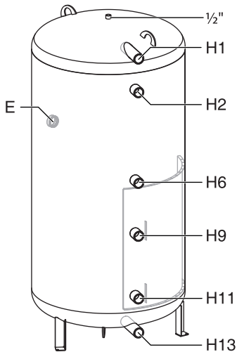
B 500, 750, 1000 300-6 ER
