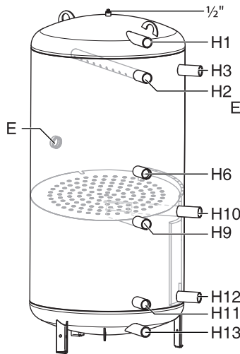
BH 500, 750, 1000-6 ERZ
